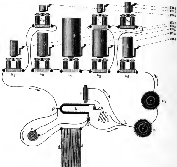
Helmholtz' Stimmgabelapparat zur Vokalsynthese.
